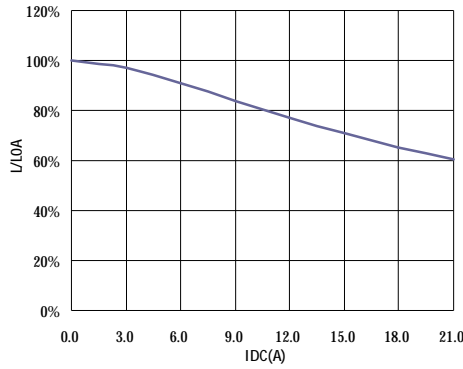
HE0618R47MS□
